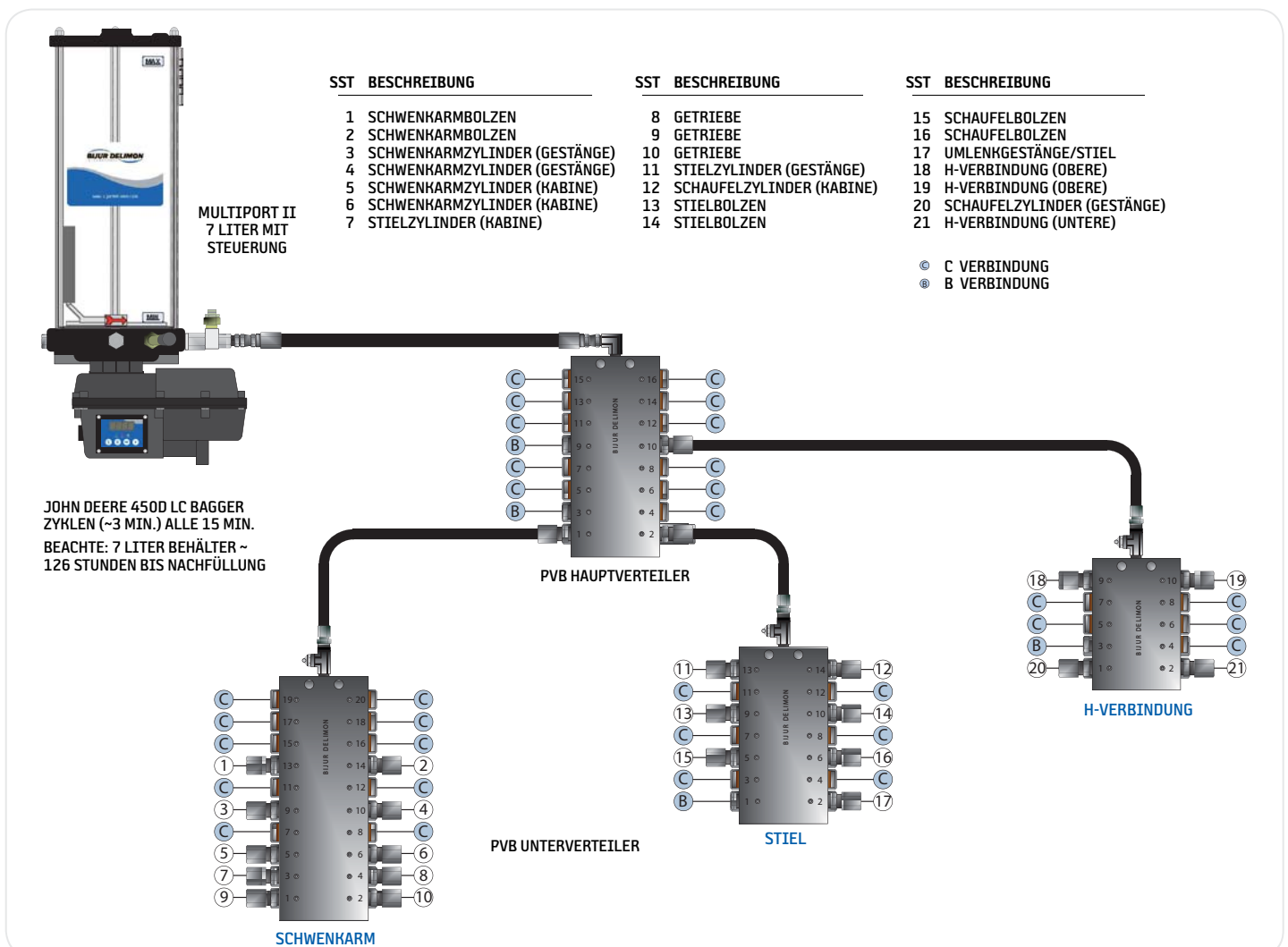
PVB Verteiler
